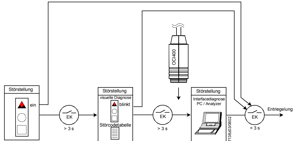
Störcodetabelle der mehrfarbigen Signalleuchte (LED)
